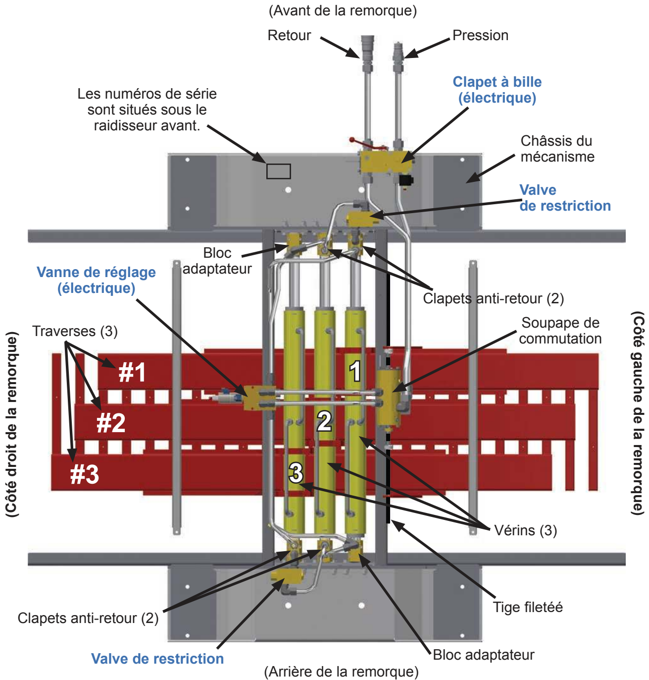
Vue du dessous de la remorque
