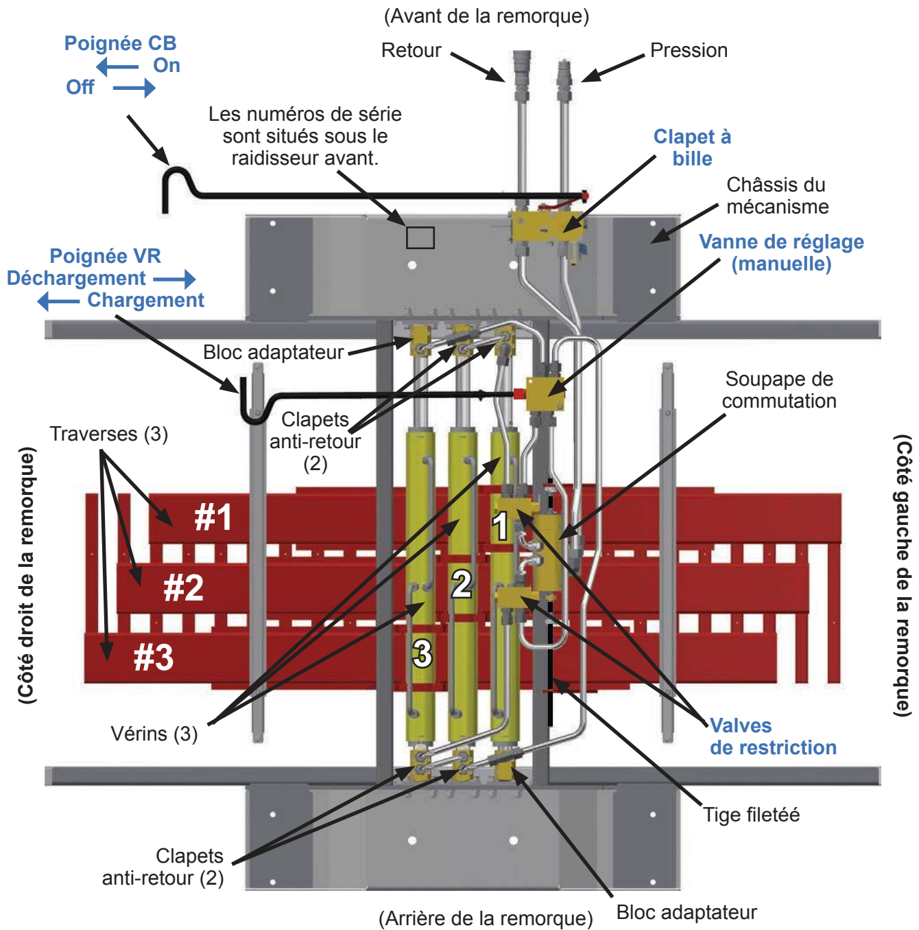
Vue du dessous de la remorque
