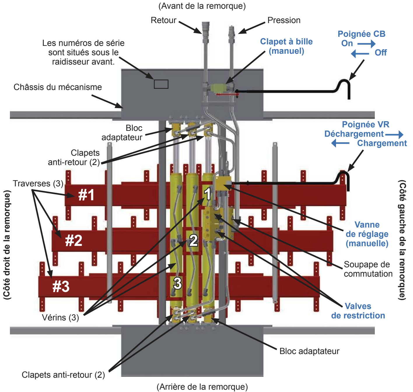
Vue du dessous de la remorque
