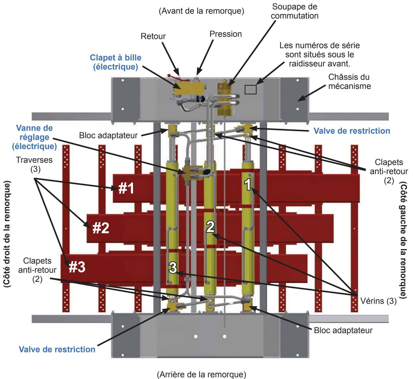
Vue du dessous de la remorque
